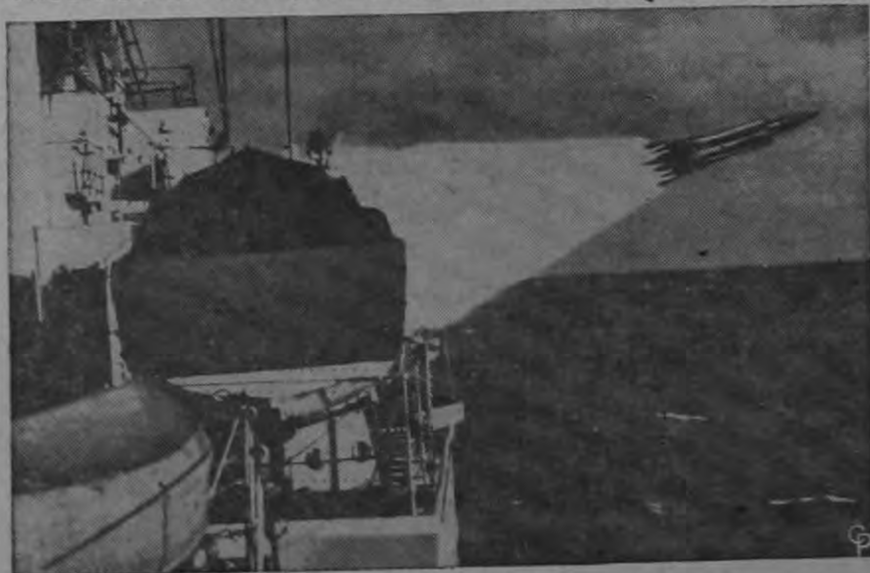
Un proyectil de prueba es disparado desde el buque de guerra Girdle Ness para pruebas de proyectiles dirigidos, durante unas recientes prácticas en el mar. El "Sea Slug" un arma británica de mediano alcance puede atacar a un avión de bombardeo enemigo a cualquier altura. El proyectil es operado y disparado desde el interior de un buque sin que personal alguno se exponga. Una triple plataforma de lanzamiento es alimentada automáticamente con el proyectil para el disparo. (INP)
